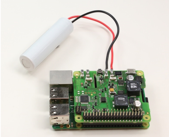
Abbildung 3.4: USV+ auf Raspberry Pi mit Akku
