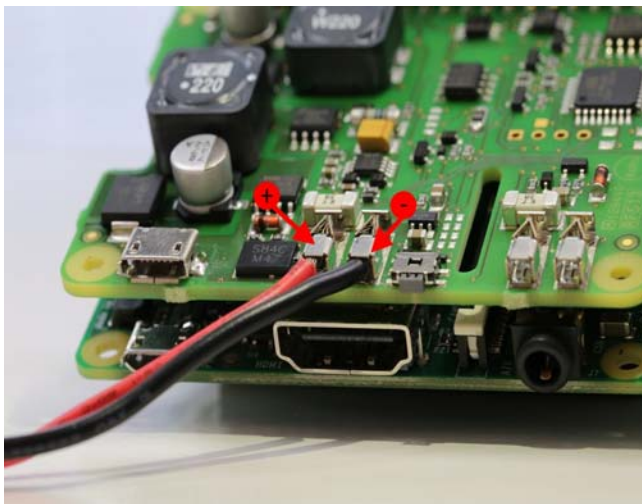
Abbildung 3.3: Anschluss Akku
