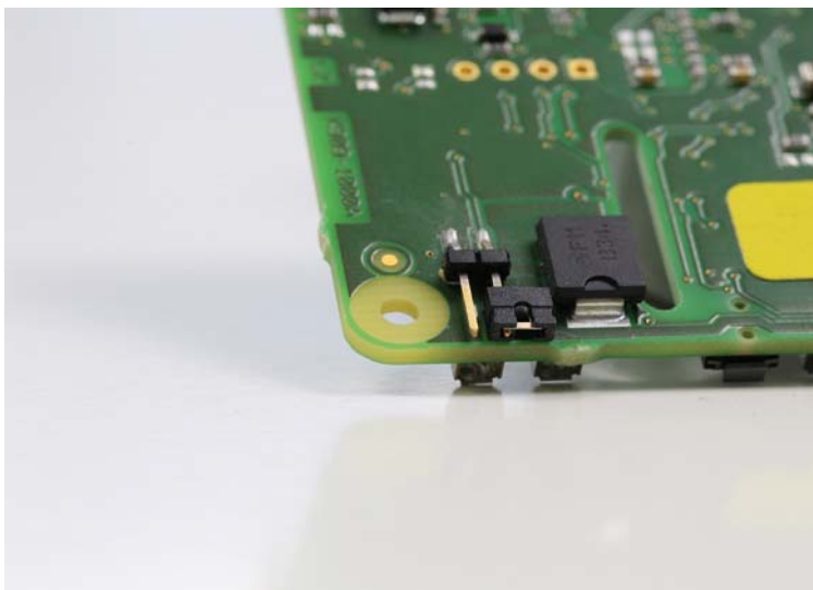
Abbildung 3.2: Jumperkonfiguration automatischer Start
