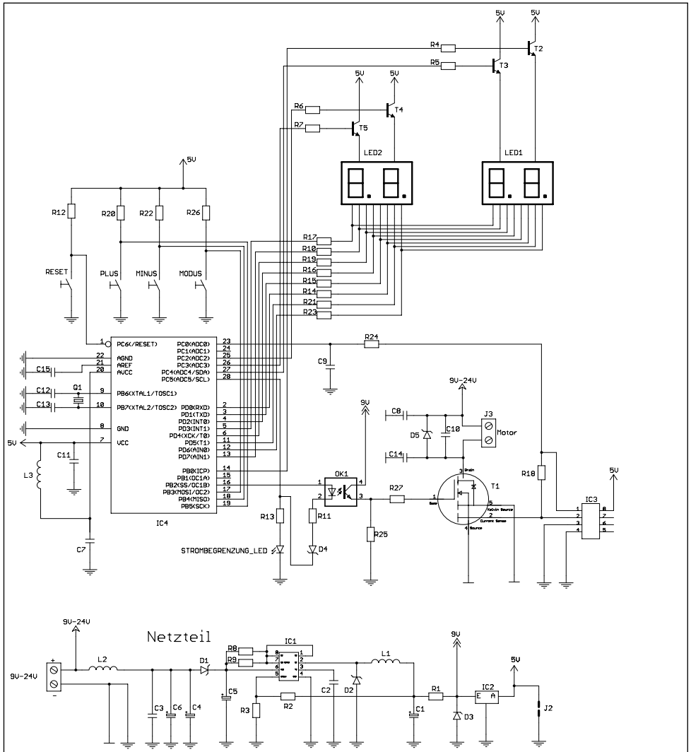
Schaltplan für den Drehzahlsteller für Gleichstrommotoren
