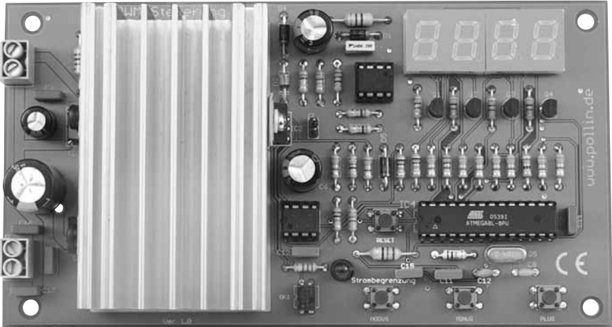
Drehzahlsteller für Gleichstrommotoren
