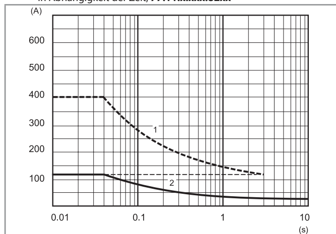
L77-11 Ausgangsbelastbarkeit - Max. Einschaltstrom (AC) in Abhängigkeit der Zeit, 77x5.x.xxx.8x50
