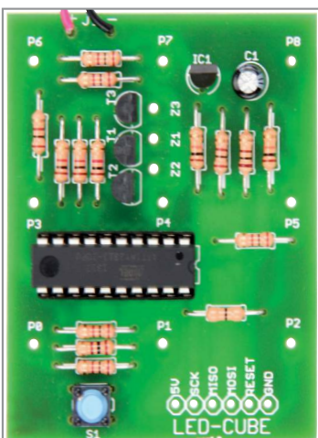
Platinenansicht (ohne LEDs)
