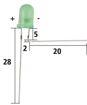
2 x LED3
