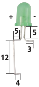
2 x LED4
