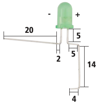
4 x LED5
