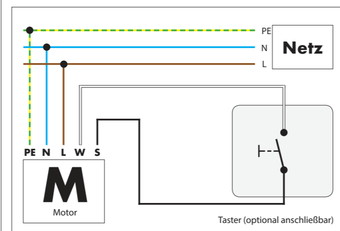
Abb.2: Anschlussschema Art. 140010 - 140050
