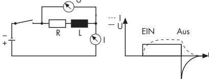
Strom- Spannungsverlauf beim Schalten einer Relaispule Abb.2
